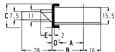
U-förmiger Stulp
