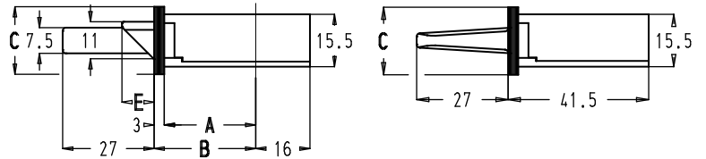
Flacher Stulp
